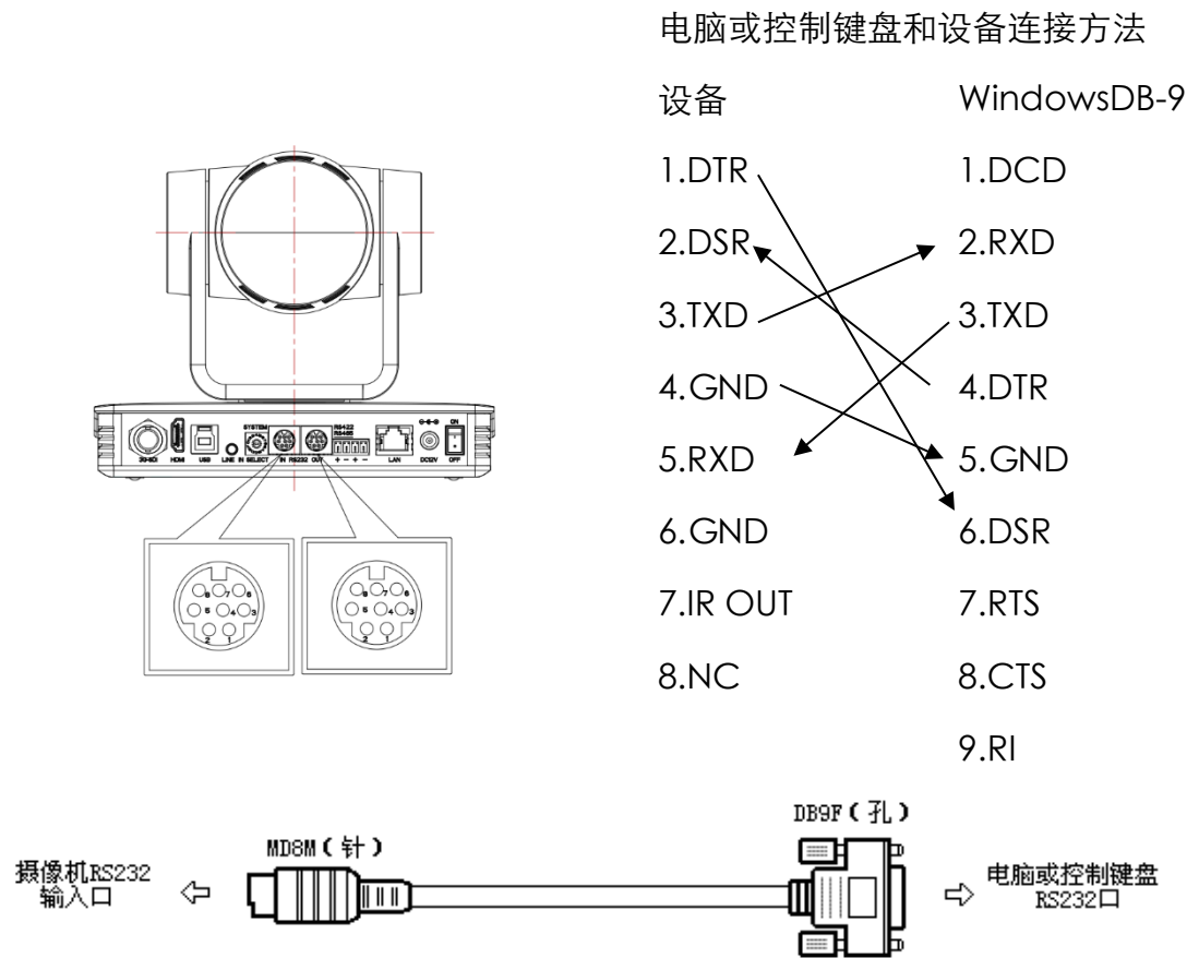
图 2-3 RS-232 接口示意图
