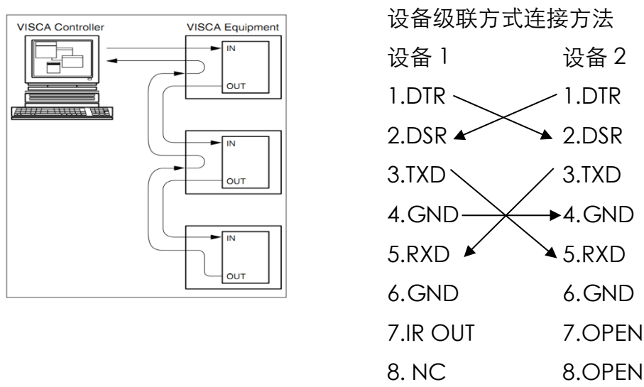
图 2-4 VISCA 组网方式示意图
