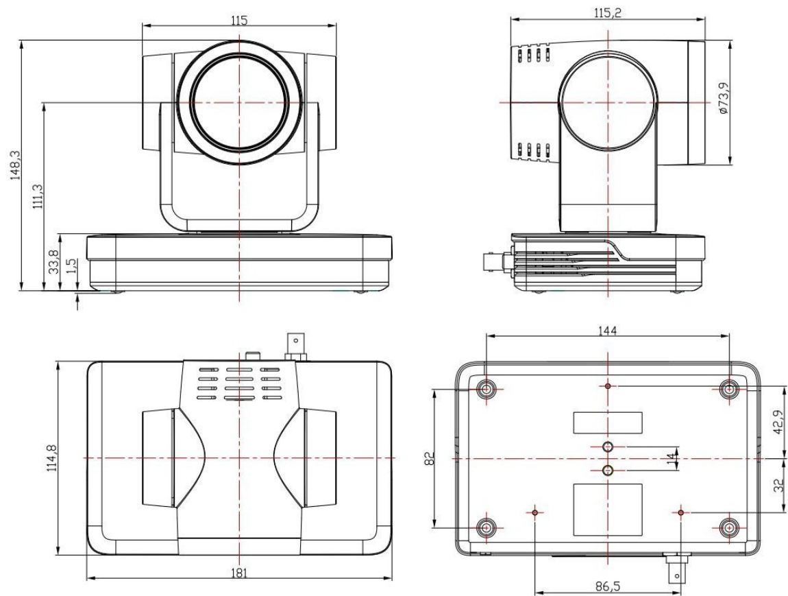
图 2-1 外型尺寸
