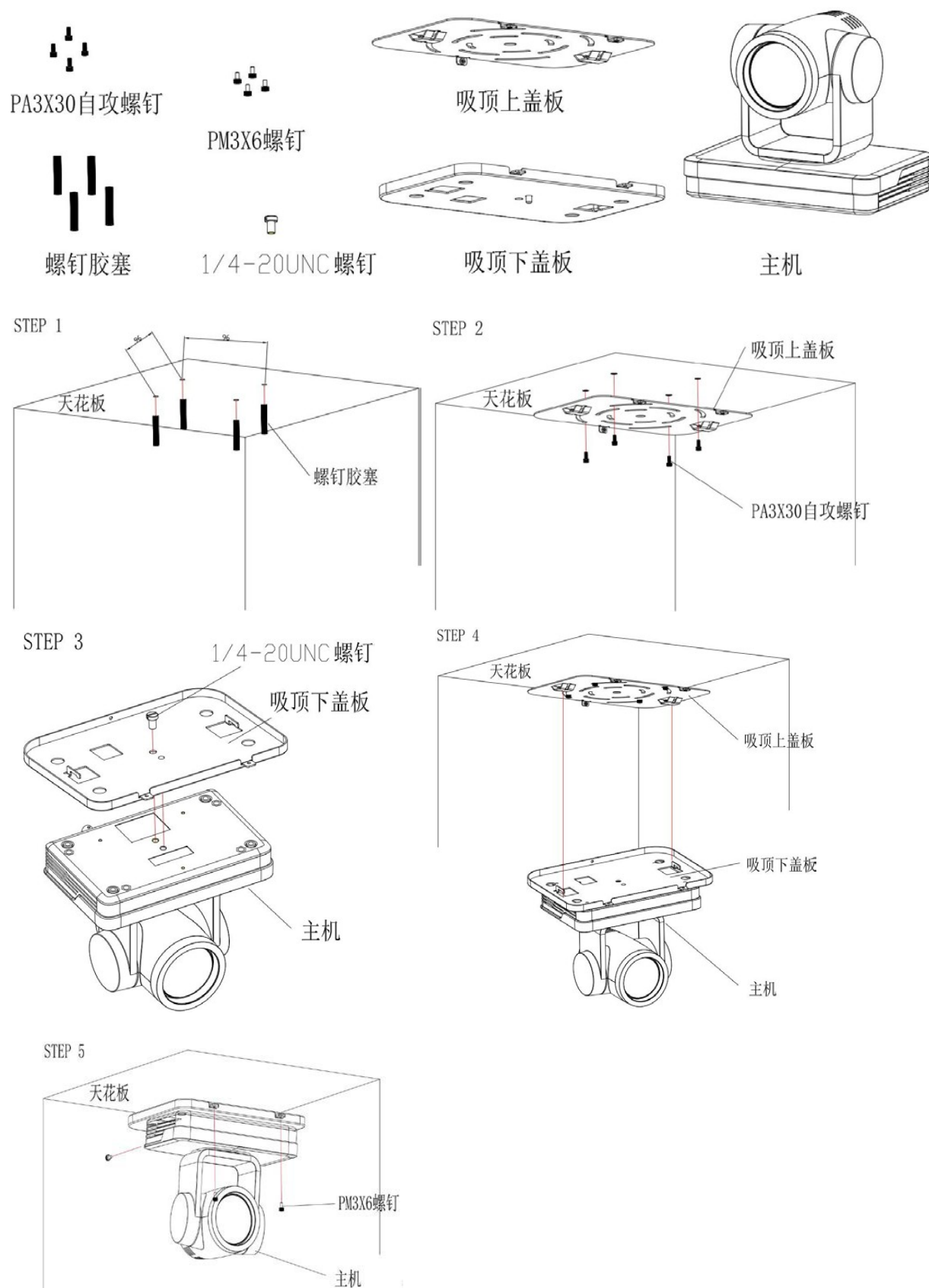
图1-3 支架倒装步骤
